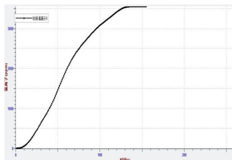
图 3 氯离子传感器测得的图像
